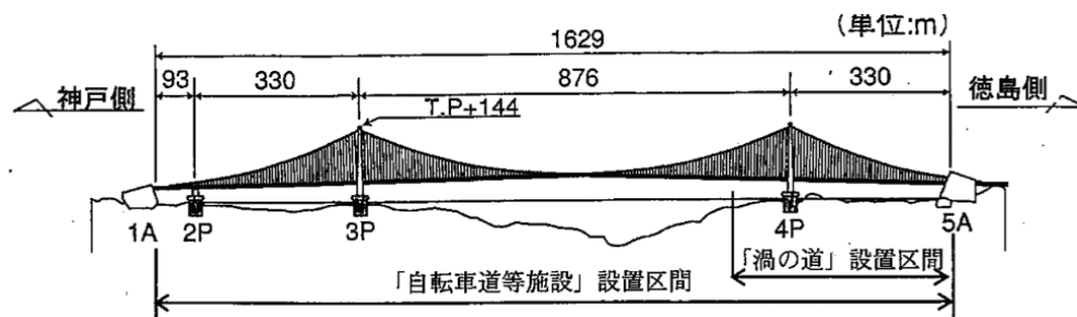
【自転車道設置イメージ(断面図)】
